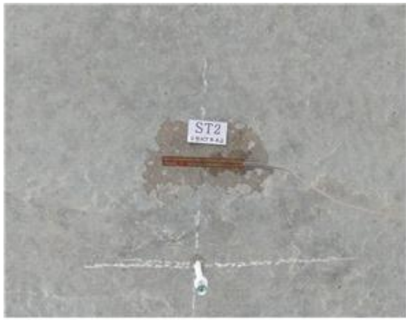
변형률계 설치 현황
