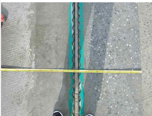
신축 유간거리 측정전경
